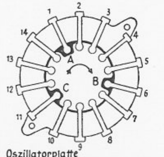
Oszillatorplatte Gezeichnete Schalterstellung: „kurz“
